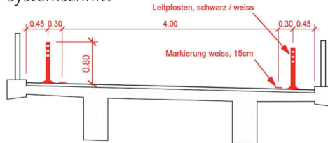
Systemschnitt
