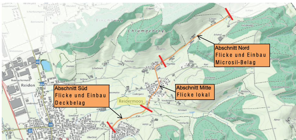
Plan Situation Übersicht bauliche Massnahmen
