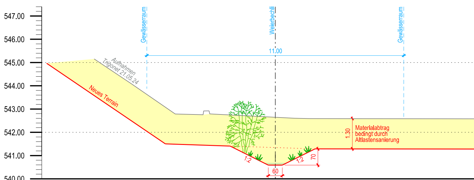
Querprofil 930 1:100
