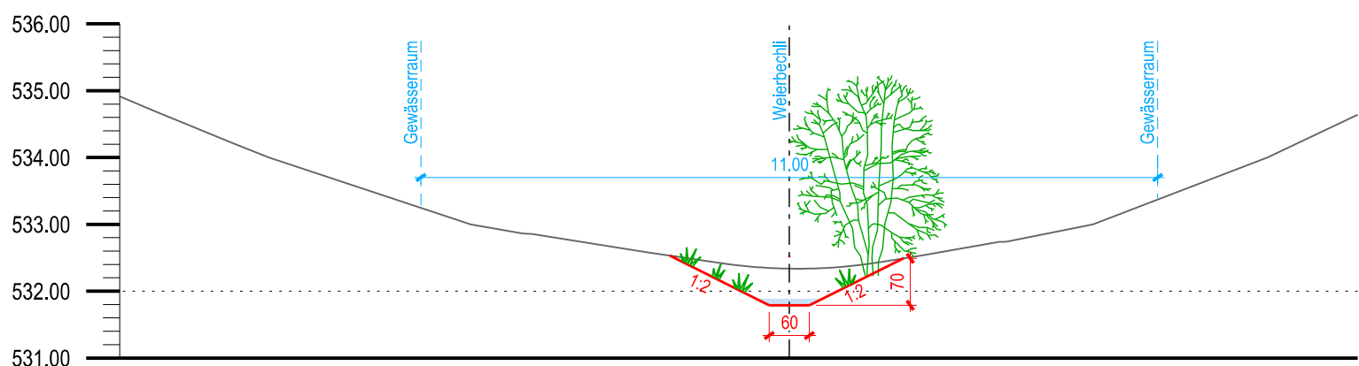
Querprofil 860 1:100
